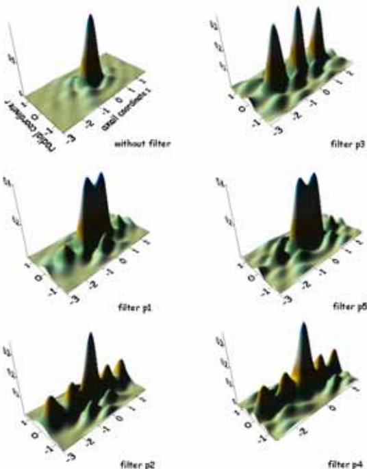
Abb.2 3D-PSF für die Filter mit nur einem Phasenring
